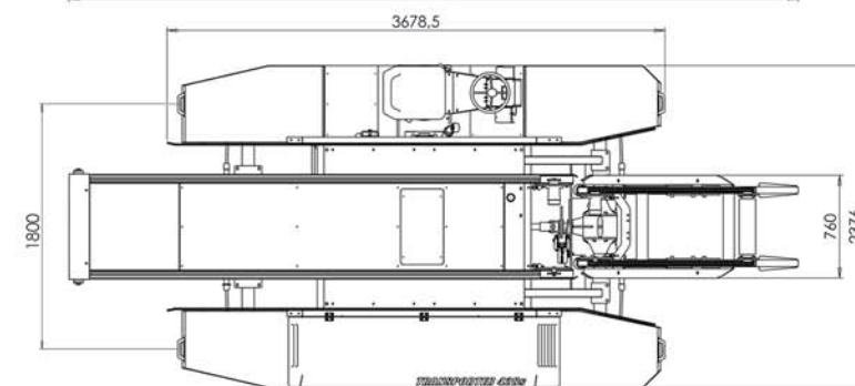
POSIZIONI DI STERZATA - STEERING POSITIONS
