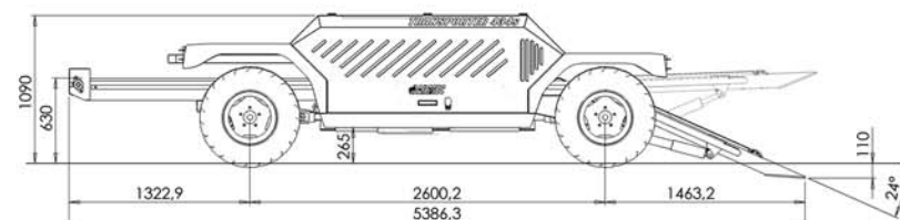
VERSIONE CON MOTORE ISUZU - VERSION WITH ISUZU ENGINE
