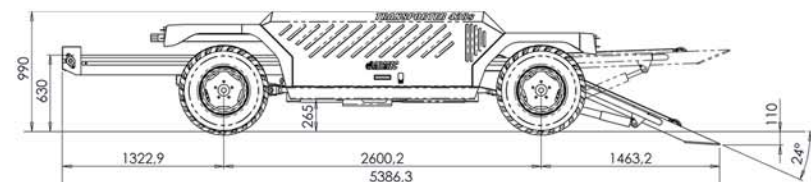
VERSIONE CON MOTORE ISUZU - VERSION WITH ISUZU ENGINE
